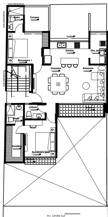
PRIMER NIVEL Superficie construida: 106.64 m 2
