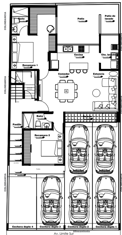
PLANTA BAJA Superficie construida: 123.75 m 2
