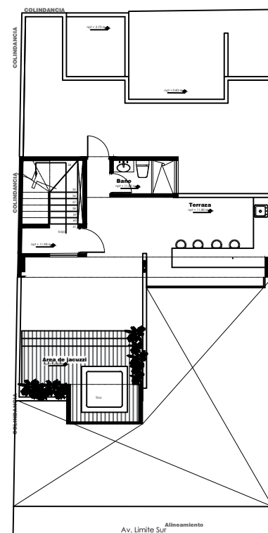
ROOF GARDEN Superficie construida: 29.04 m 2
