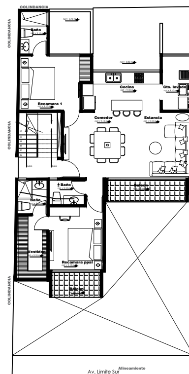
TERCER NIVEL Superficie construida: 109.06 m 2
