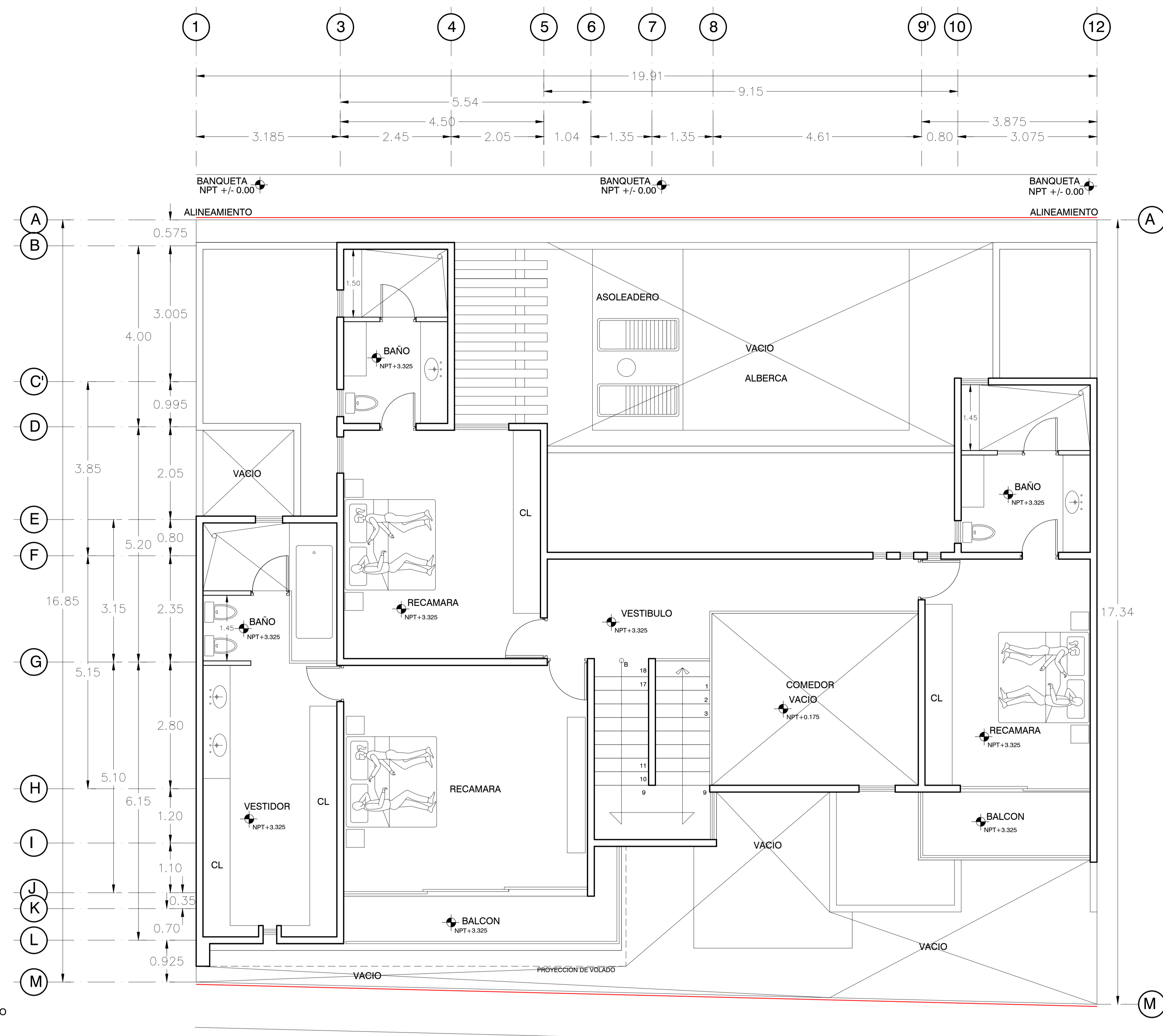
PLANTA ALTA
